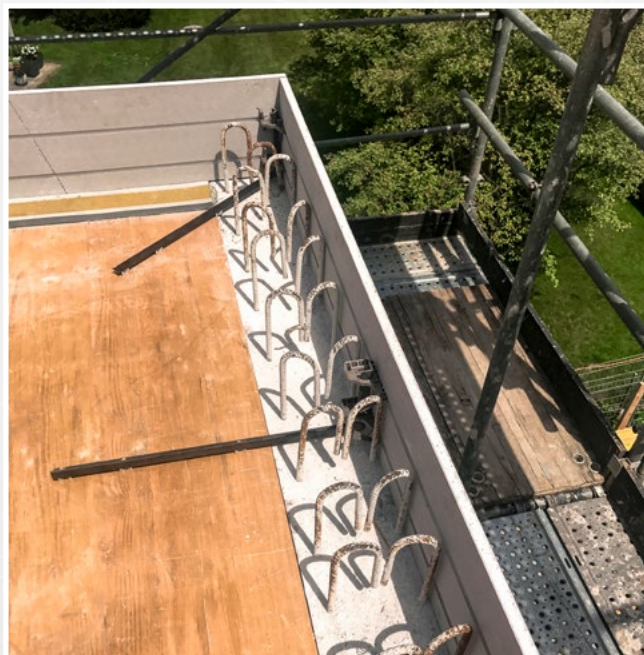
Die Winkel können horizontal stufenlos verschoben werden um z.B. Anschlusseisen, Gleitlagern und Einlagen auszuweichen.
