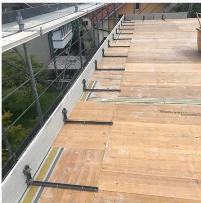
Zum Fixieren des 2.8 m langen Bordfix Elements werden die Deckenwinkel ausgeklappt, das Element an den Deckenrand geschoben und mit Aluminium-Nägeln fixiert
