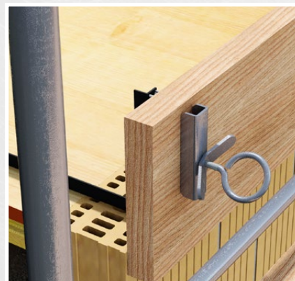
Fixation avec papillon Randfix
