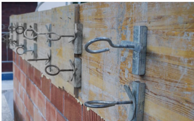
Deux papillons sont nécessaires avec l'équerre Randfix, art. 1105.
