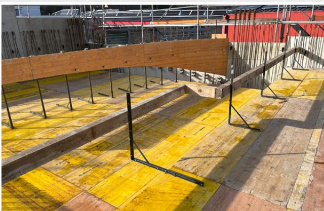
Randfix convient également pour le coffrage des décrochements
