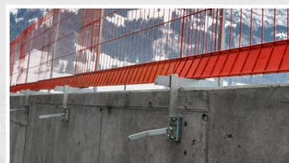
Pince Kombifix avec protection latérale Safe-Gard comme protection contre les chutes
