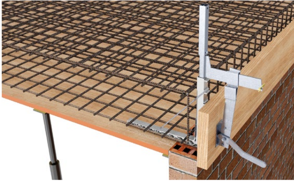
Équerre Kombifix Maxi avec pince Kombifix universelle sans barrière de sécurité
