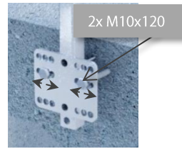
Fixation de montant, quadrangulaire
