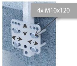
Fixation de montant, quadrangulaire
