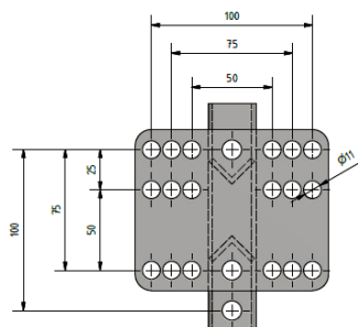
Gabarit de perçage montants ProSide
