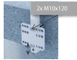
Fixation de montant, verticale
