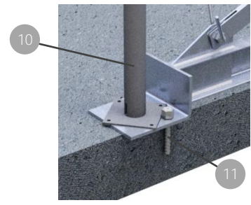
Befestigungsvariante 1 mit 1 Deckenstütze + Befestigung pro Tragholmen
