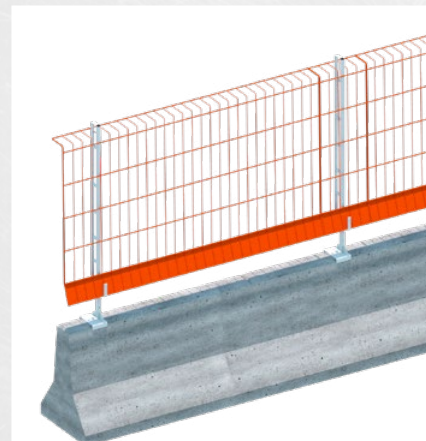
Safe-Gard Seitenschutz montiert auf dem New Jersey Element
