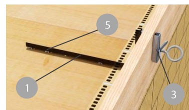
System Randfix bei Deckenschalung aus Holz.
