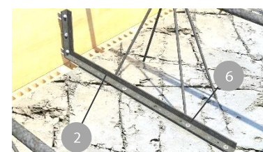
System Randfix mit Elementdecken und Nageldübel.
