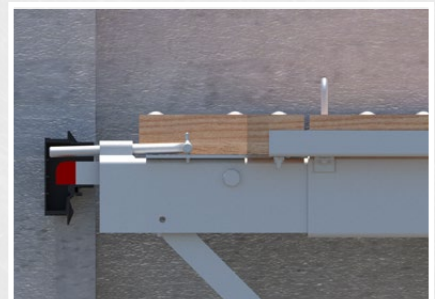
...und automatisch in die einbetonierten «BKA Aussparungen Breit» einhängen.
