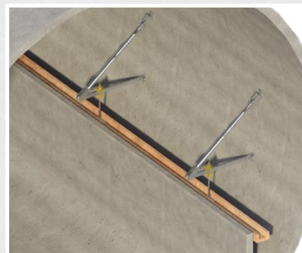
Der Einlagehalter dient zum Halten von Einlagen z.B. bei Tunnelbauten
