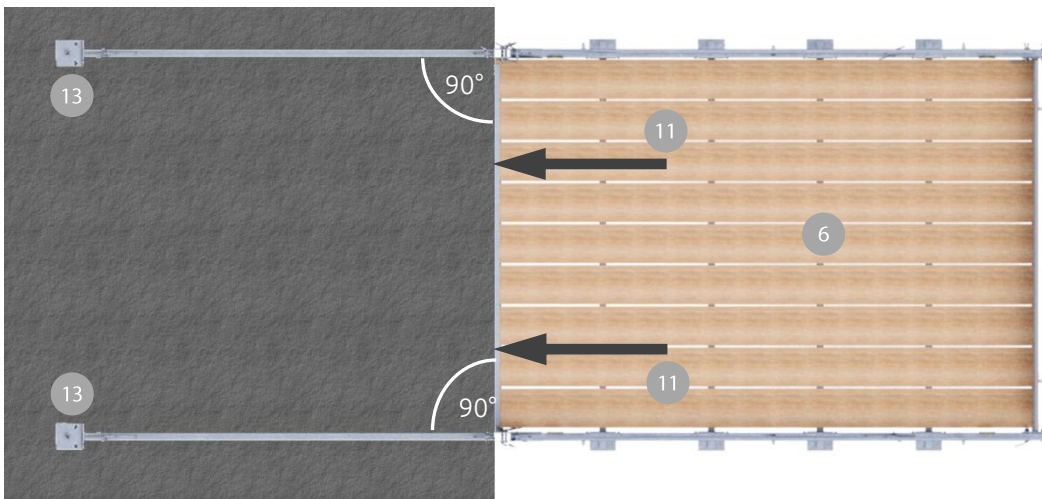
Befestigungsvariante 1 mit 1 Deckenstütze + Befestigung pro Tragholmen
