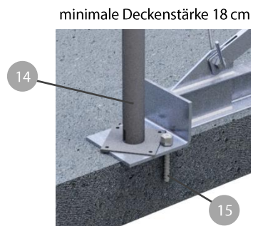
Befestigungsvariante 1 mit 1 Deckenstütze + Befestigung pro Tragholmen
