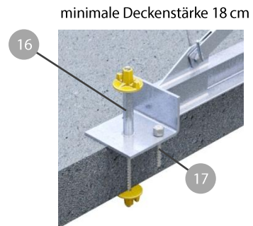
Befestigungsvariante 2 mit 1 DW-Stab+ Befestigung pro Tragholmen
