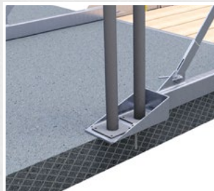
Befestigung mit 2 Deckenstützen und einem Anker
