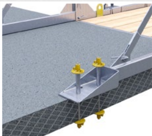
Befestigung mit 2 DW-Stäben
