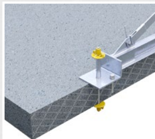
Befestigung mit einem DW-Stab und einem Anker
